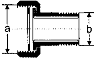
Рис. 3. Внешнее резьбовое соединение
